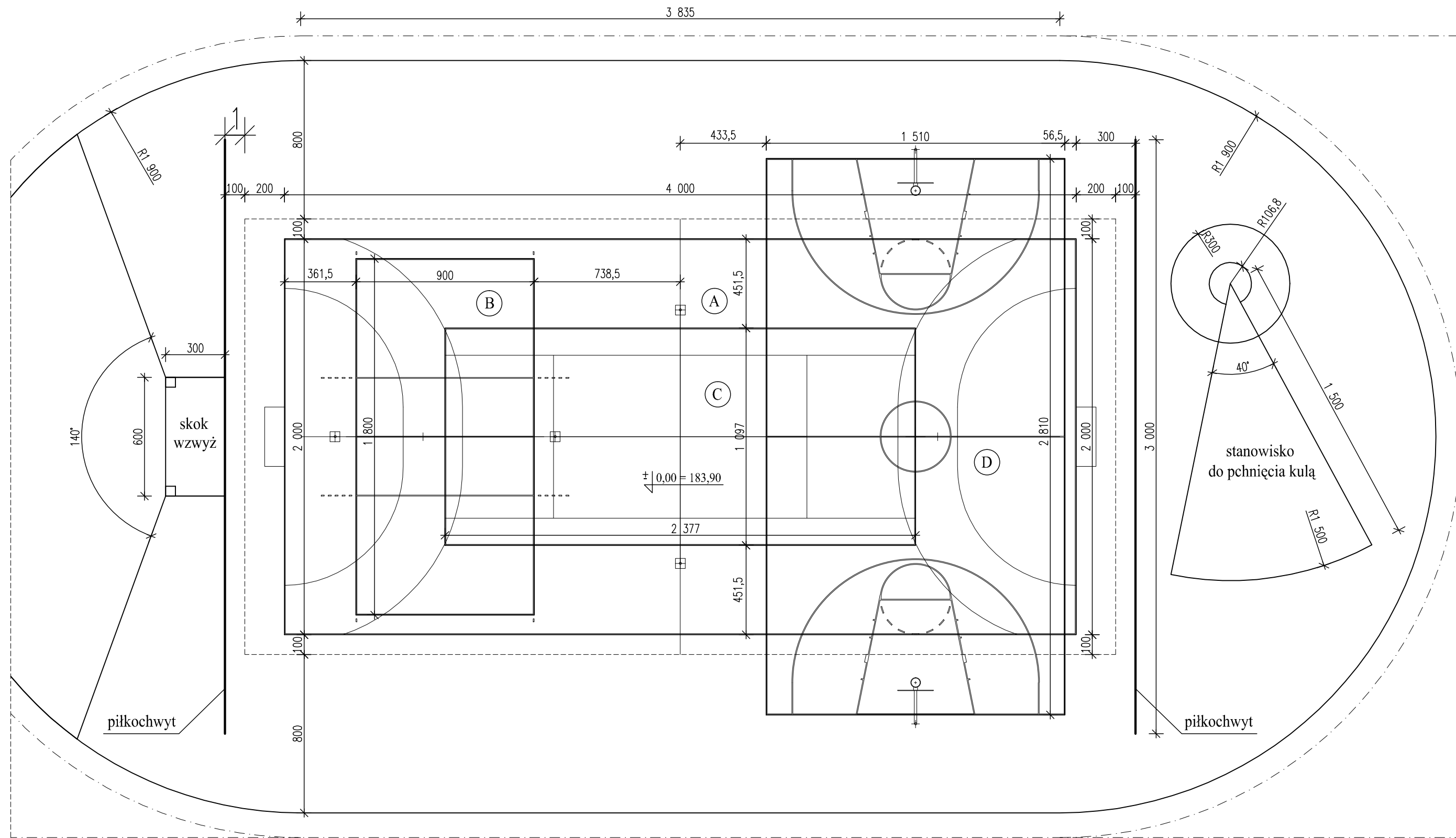
RZUT BOISKA WIELOFUNKCYJNEGO SKALA 1:200
