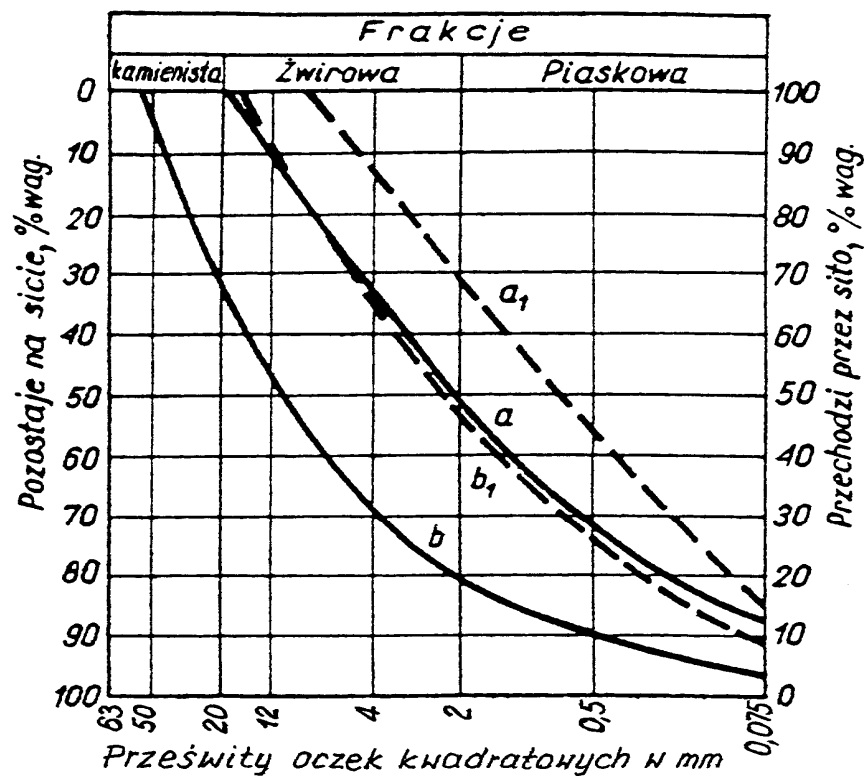
Rysunek 1. Obszar uziarnienia optymalnych mieszank żwirowych
